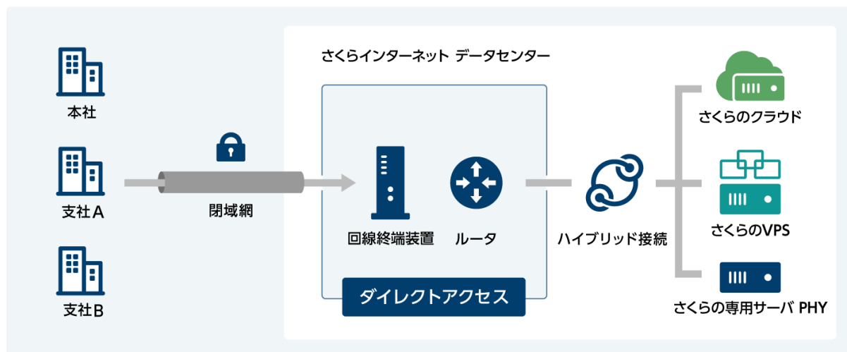
ダイレクトアクセスを利用した閉域網と当社のホスティングサービス接続の概念図
