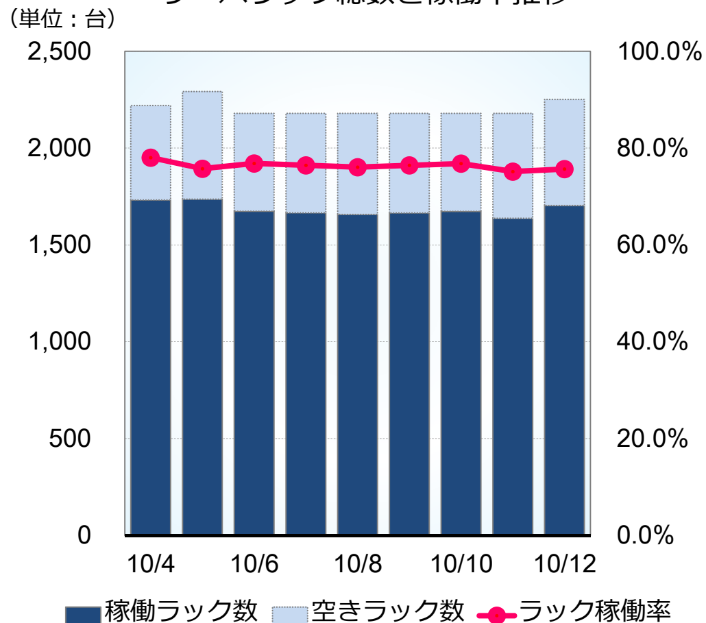
サーバラック総数と稼働率推移
