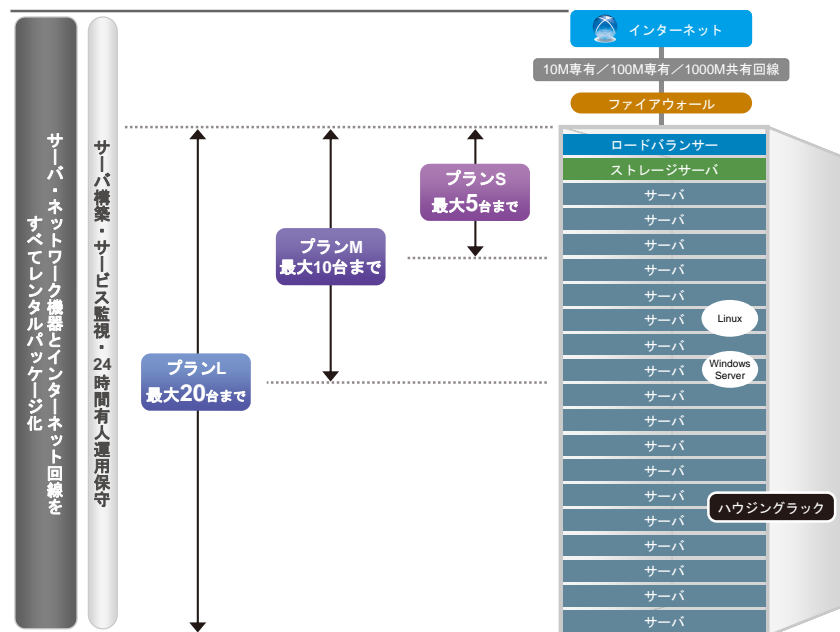
専用サーバ Platform St のサービス構成イメージ
